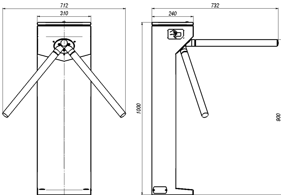
Рис.6Б Турникет. Габаритные размеры
