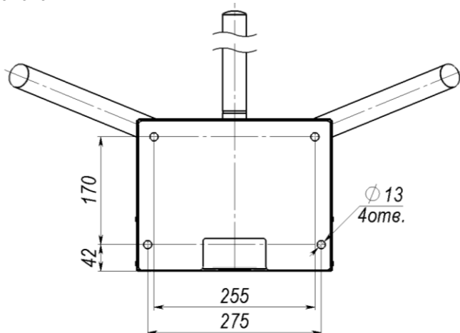
Рис.6А Основание турникета. Вид снизу.
