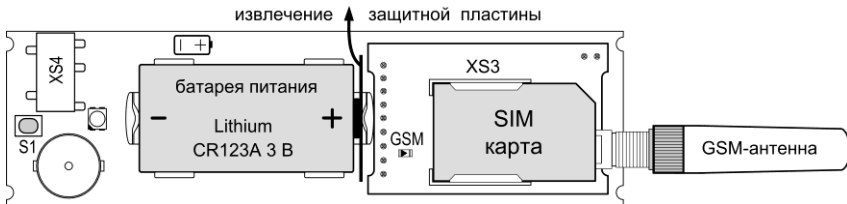
Рис.6 Установка SIM-карты, извлечение защитной пластины, подключение внешней GSM-антенны (только для варианта 2)
