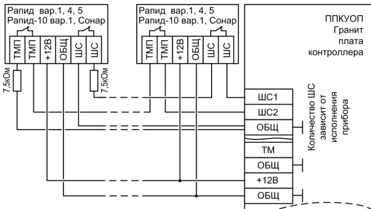
Рис.Б3 Схема подключения охранных извещателей Рапид вар.1,4,5, Рапид-10 вар.1, Сонар (тампер подключён к отдельному ШС)
